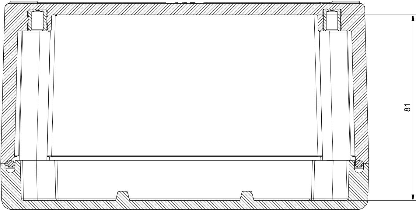
Sezione A-A
