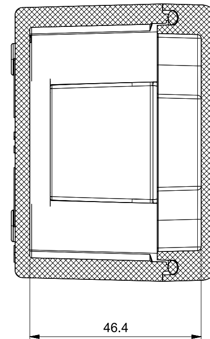
Sezione A-A
