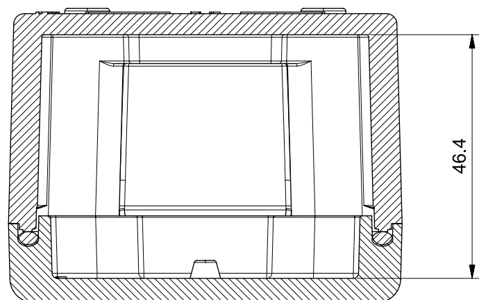
Sezione A-A
