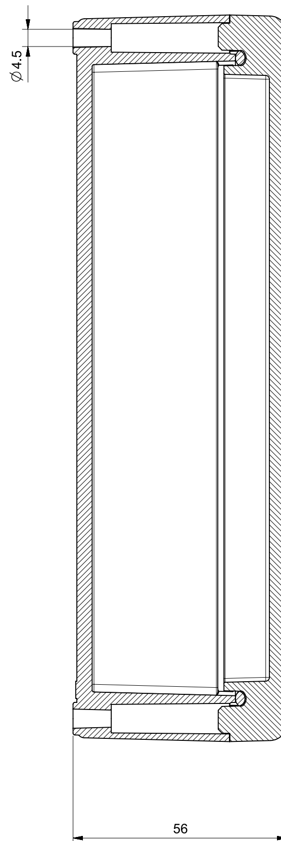
Sezione B-B
