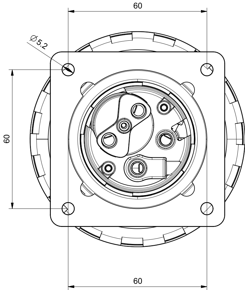
DIAMETRO DI FORATURA PANNELLO PANEL DRILLING HOLE
