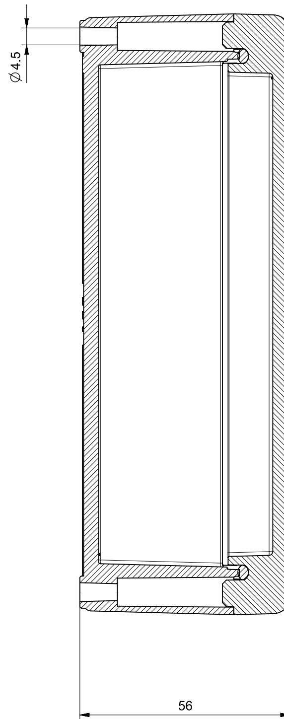
Sezione B-B
