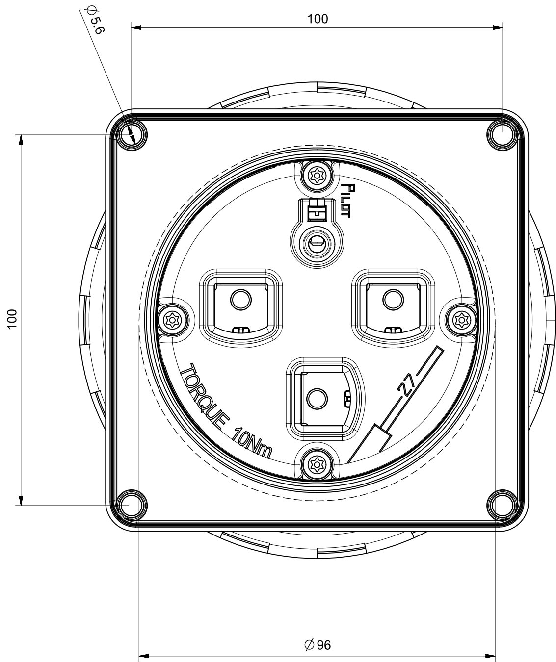
DIAMETRO DI FORATURA PANNELLO PANEL DRILLING HOLE
