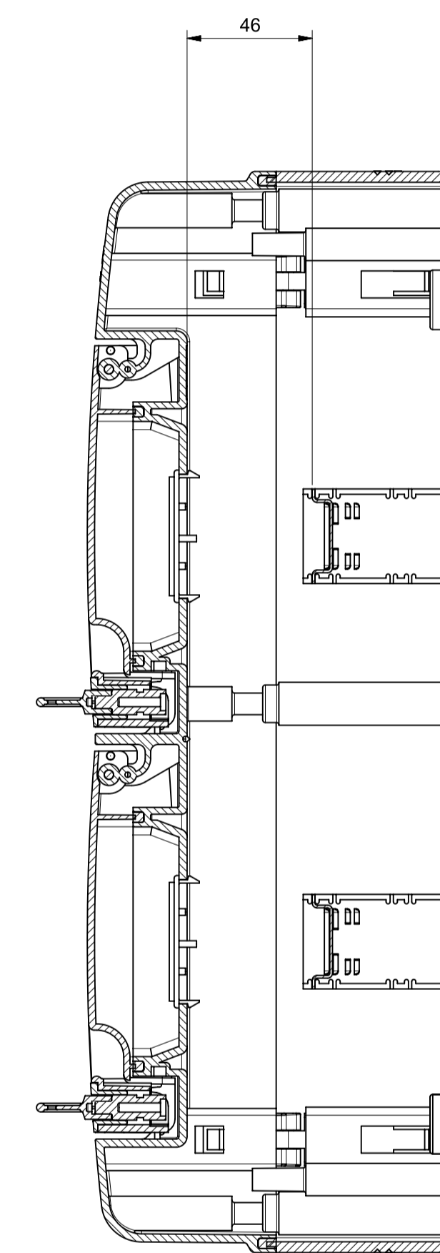
Sezione A-A
