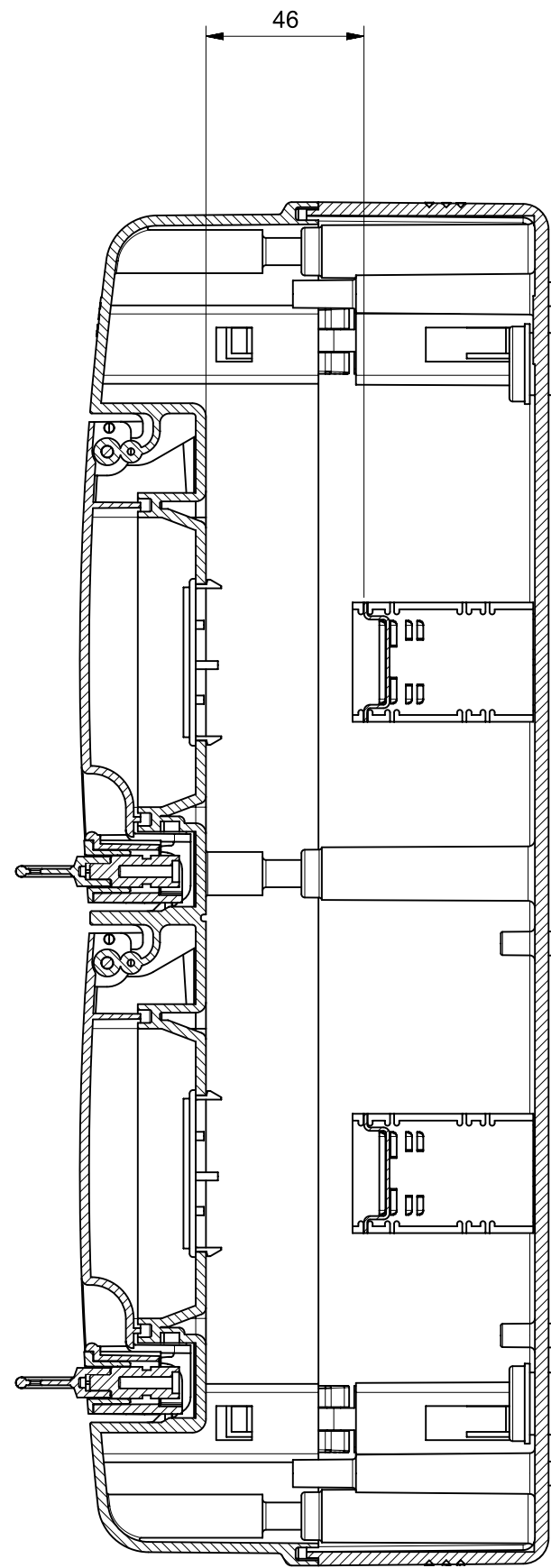
Sezione A-A
