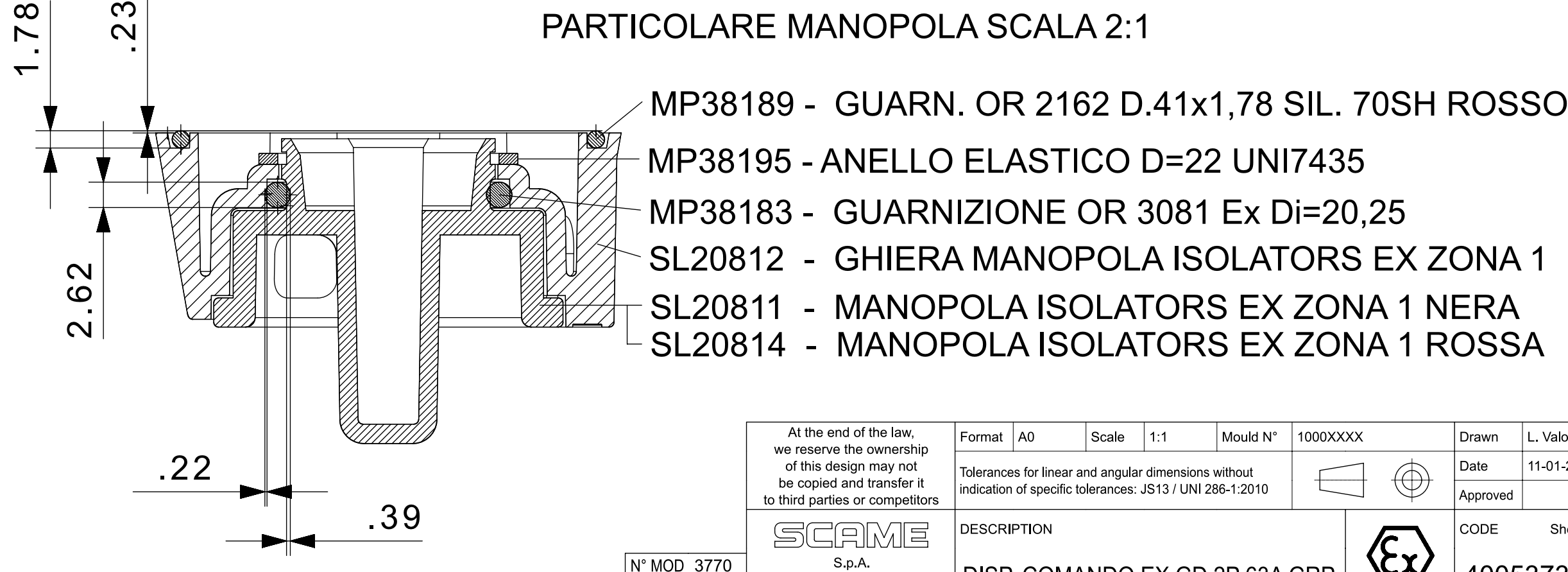
PARTICOLARE MANOPOLA SCALA 2:1
