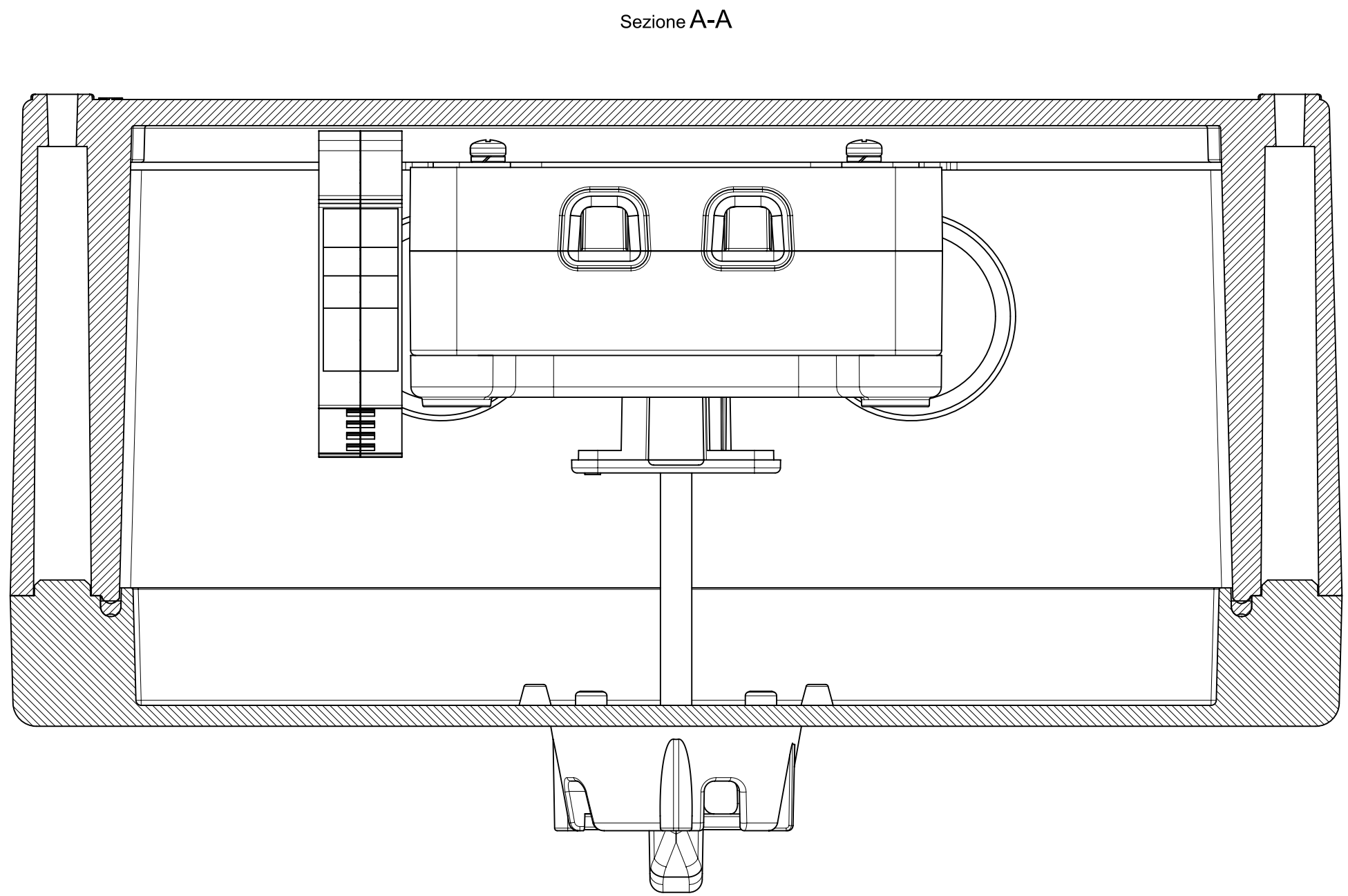
PARTICOLARE GUARNIZIONE COPERCHIO SCALA 10:1
