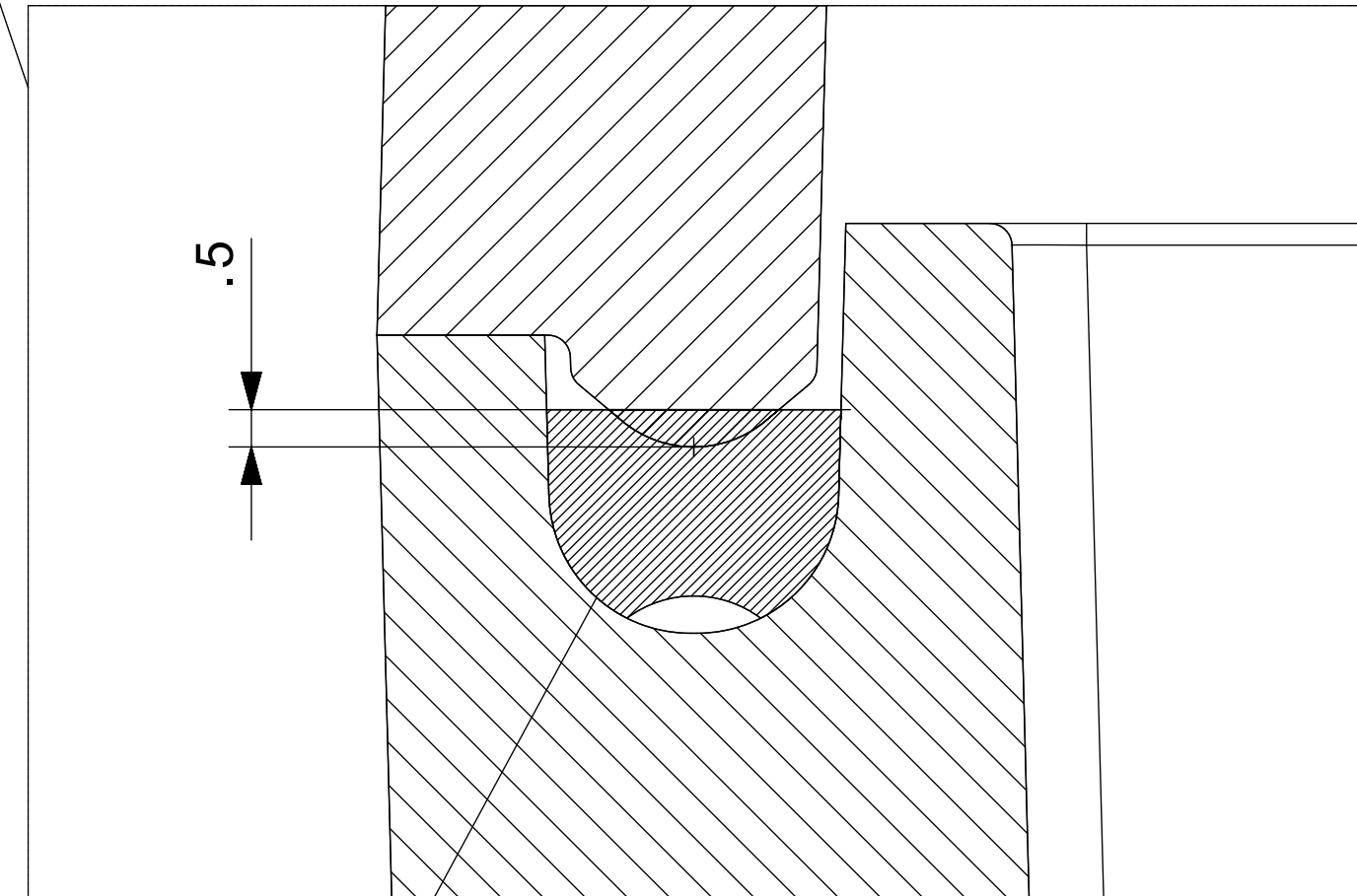
PARTICOLARE GUARNIZIONE COPERCHIO SCALA 10:1
