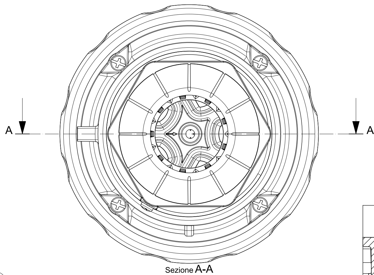
Sezione A-A
