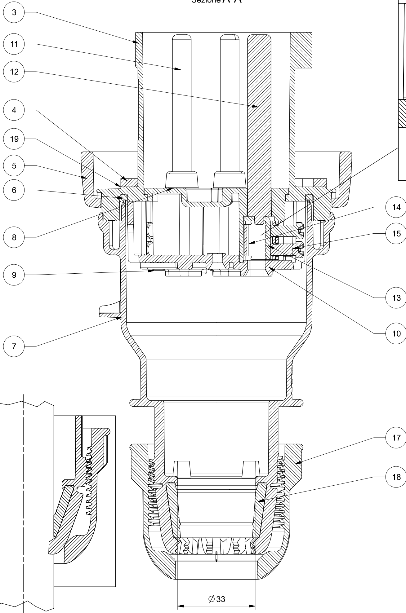
Sezione A-A
