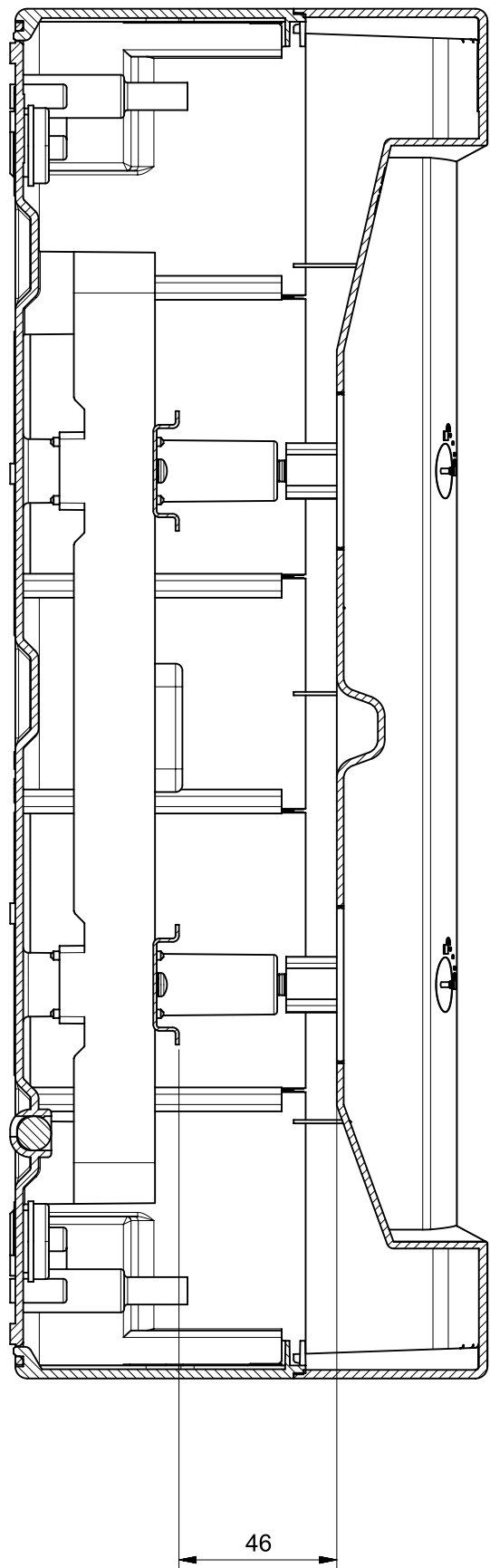
Sezione A-A
