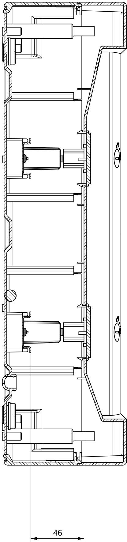
Sezione A-A
