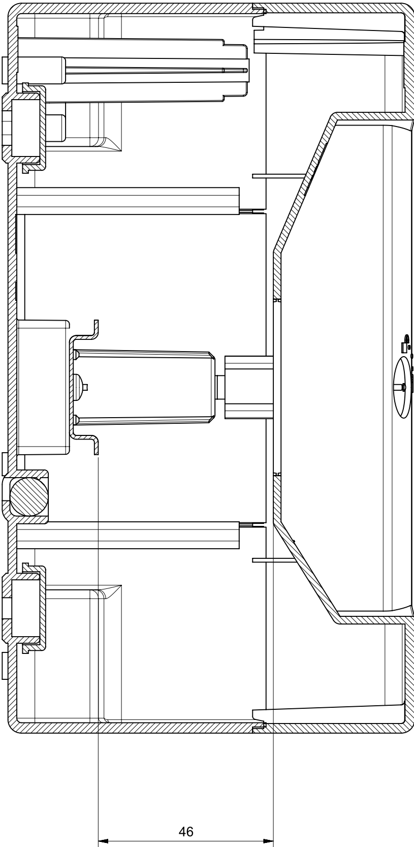
Sezione A-A
