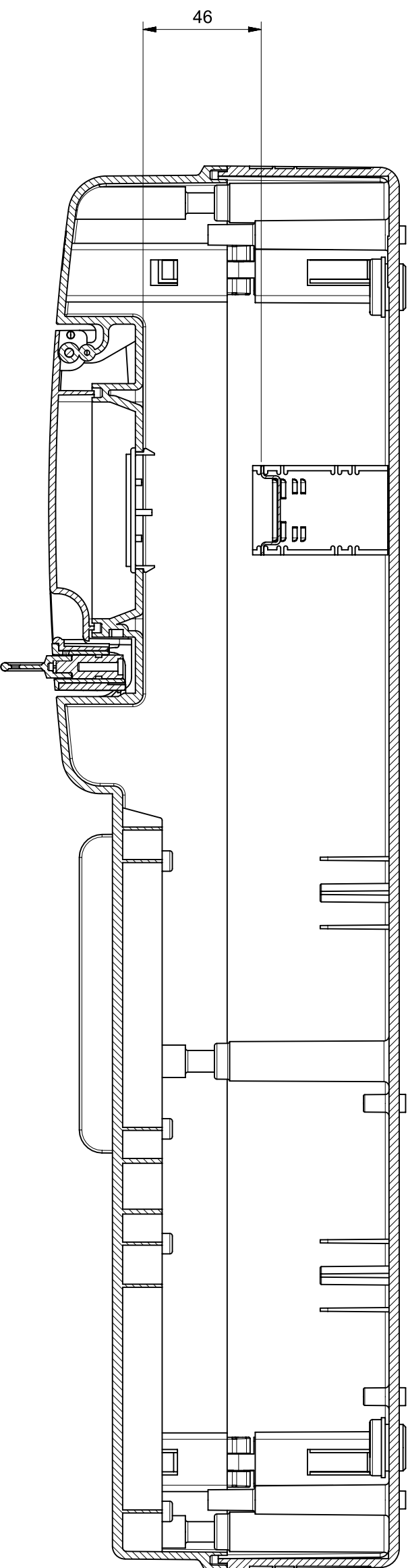
Sezione A-A
