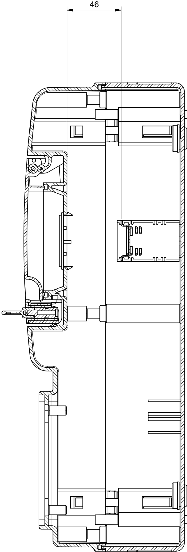
Sezione A-A
