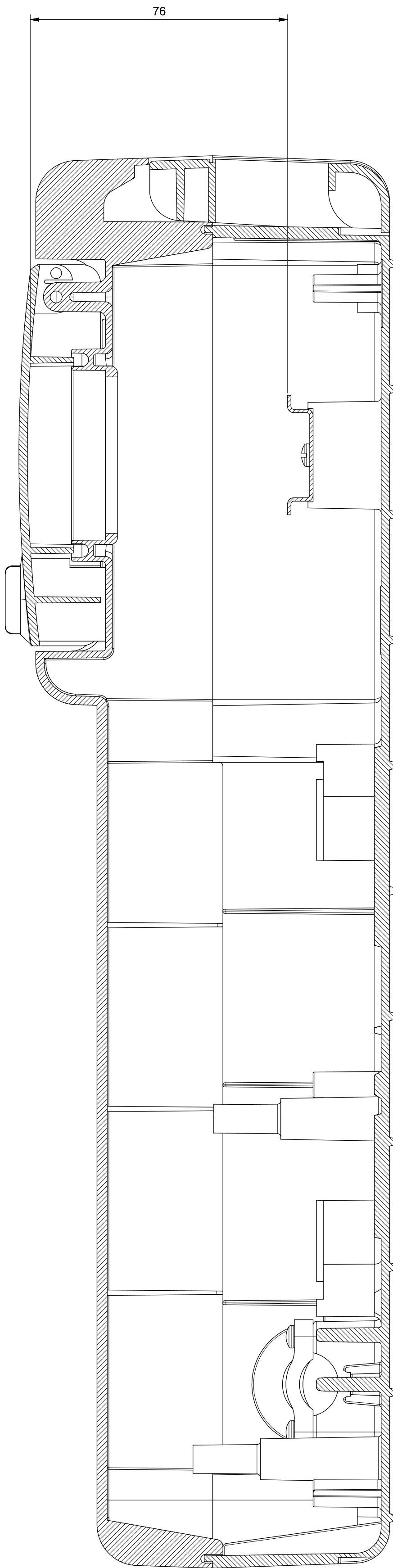
Sezione A-A
