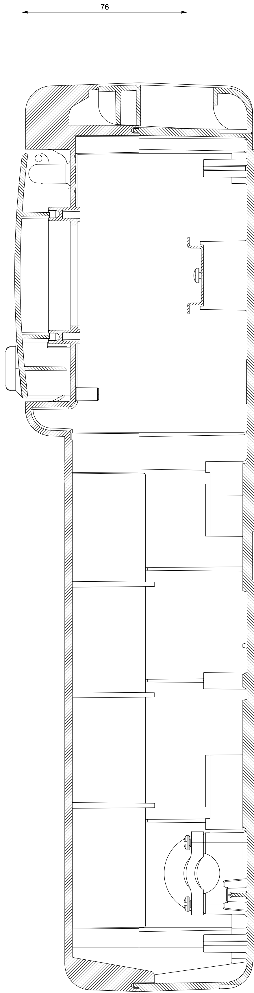
Sezione A-A
