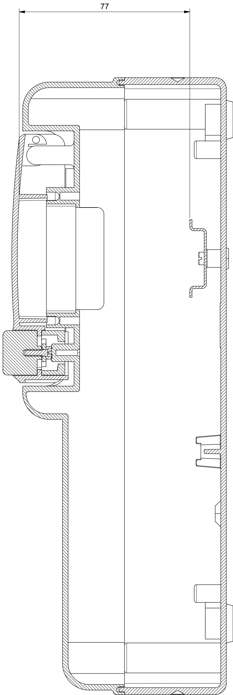
Sezione A-A
