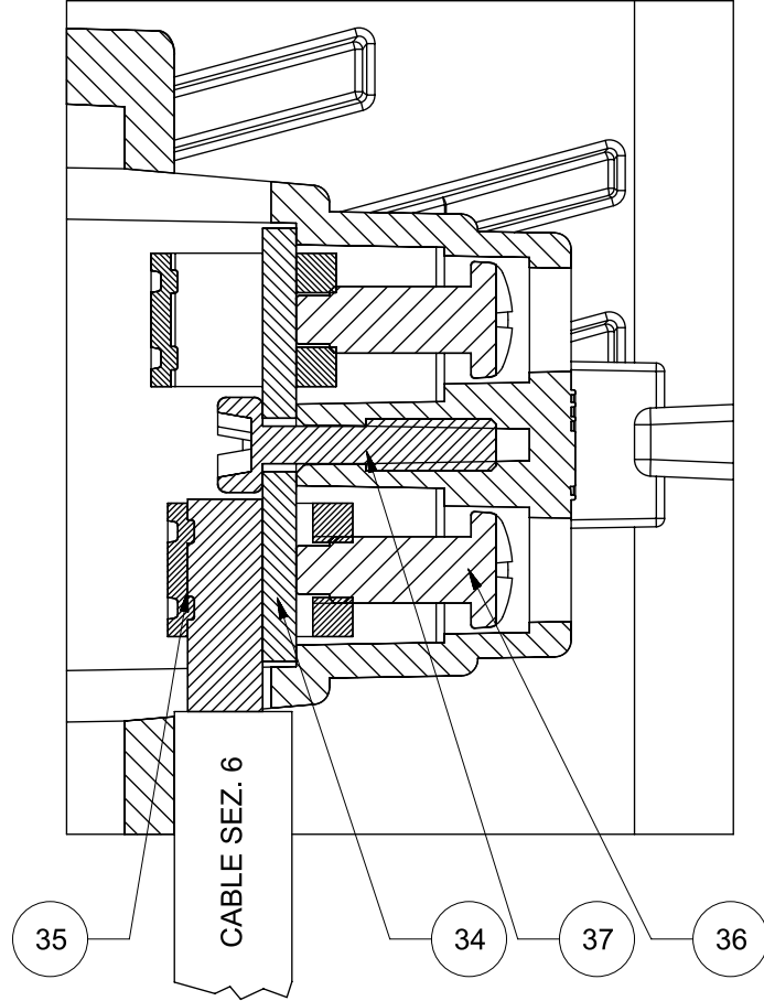
SEZIONE MORSETTO TERRA SCALA 2:1
